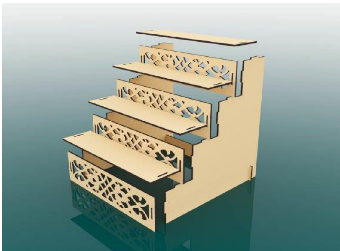
113 - 4-Shef-Display-Stand-Laser.jpg
